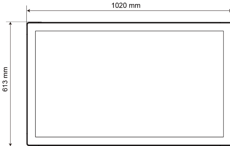
Rückseite
